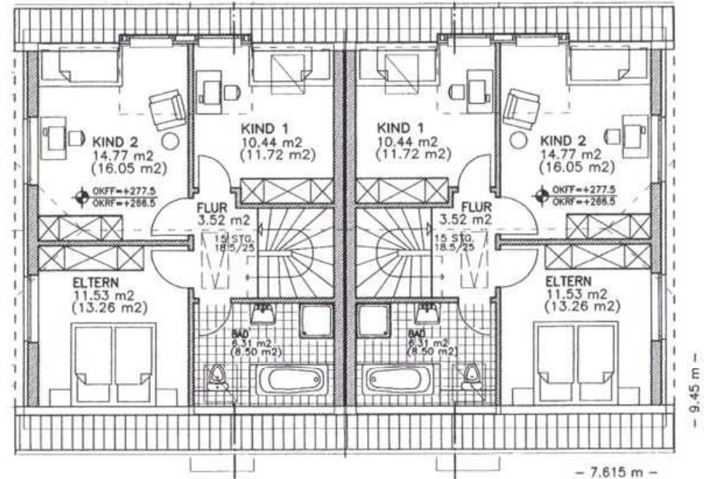
Bauherrenvariante
